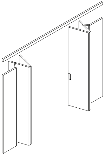
Rototraslante doppia, due ante. Double rototranslating door, two doors.
