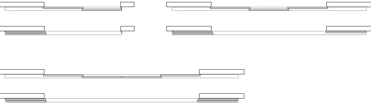
l'anta anteriore totalmente aperta trascina l'anta posteriore when fully open, the front door drags the rear door
